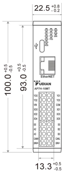
主视图
