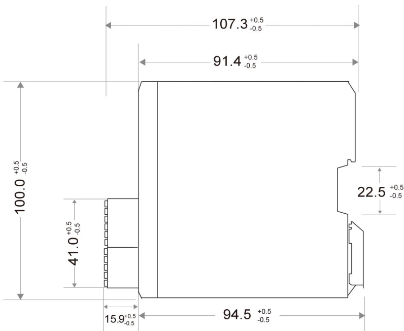
侧视图
